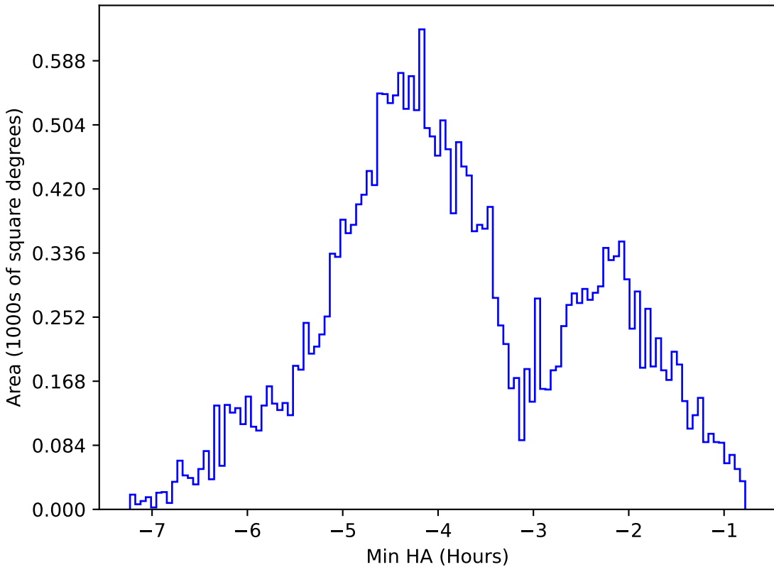
weather_cloudso2v3.4_10yrs All sky g band: Min HA
