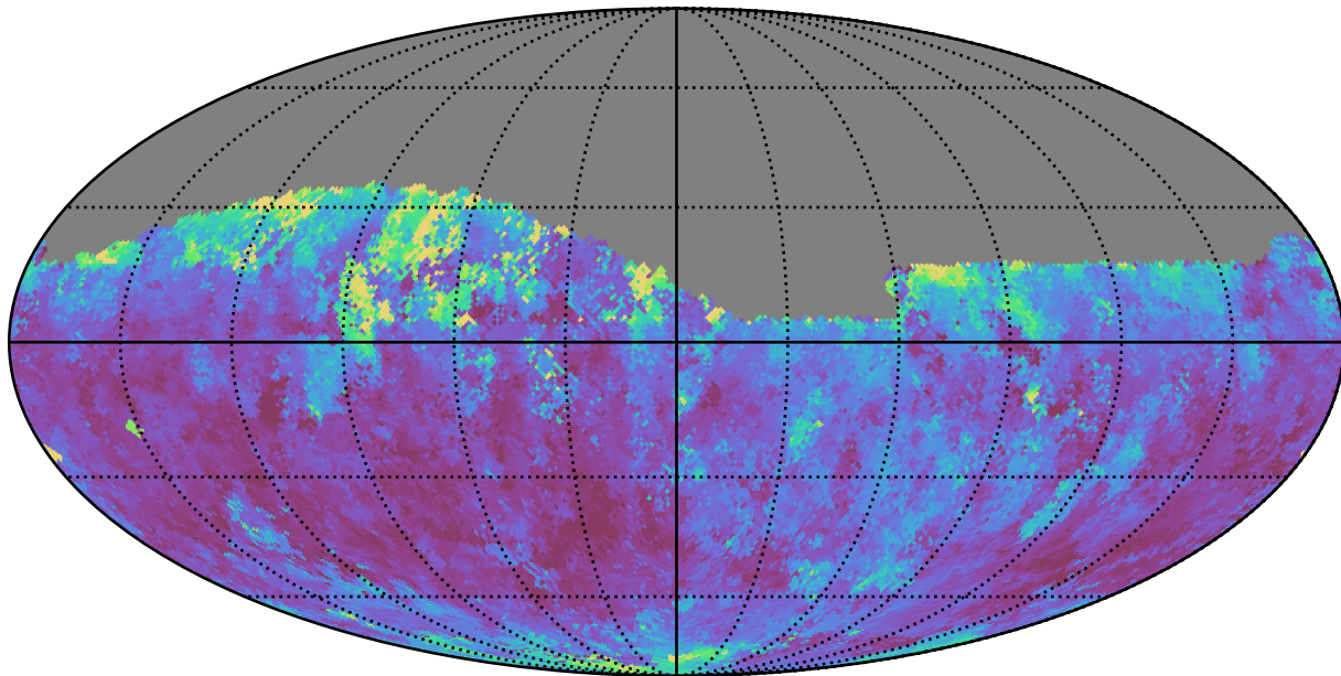
weather_cloudso2v3.4_10yrs Yr 1 z band: Median seeingGeom
