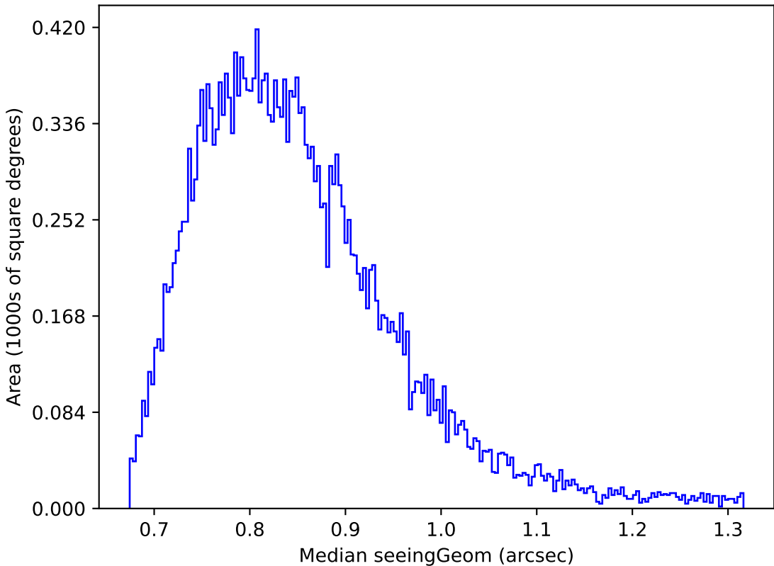
weather_cloudso2v3.4_10yrs Yr 1 z band: Median seeingGeom
