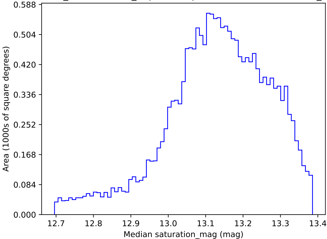
weather_cloudso2v3.4_10yrs WFD y band: Median saturation_mag
