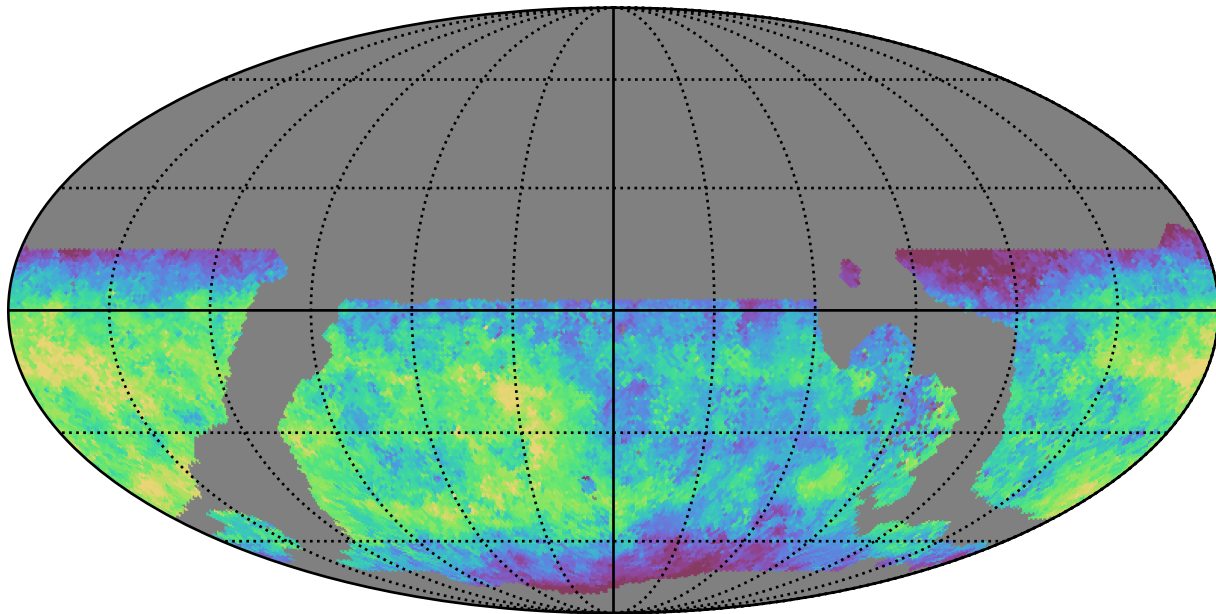
weather_cloudso2v3.4_10yrs WFD u band: Median saturation_mag
