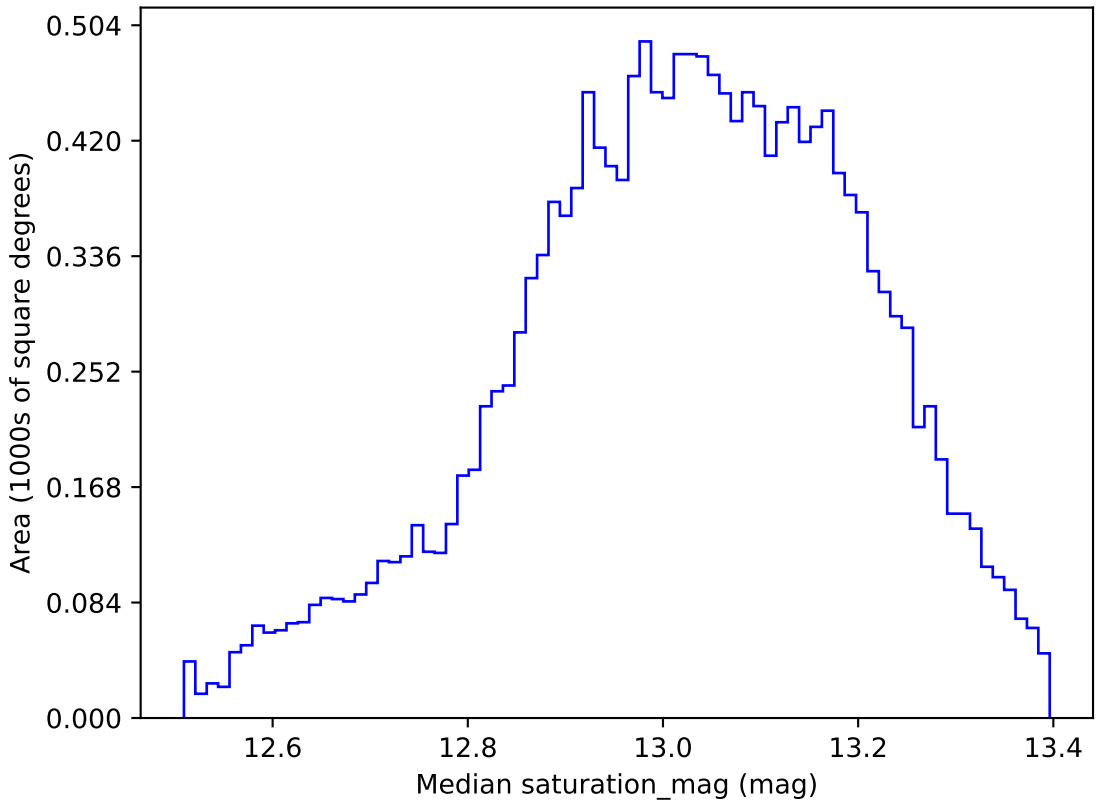
weather_cloudso2v3.4_10yrs WFD u band: Median saturation_mag
