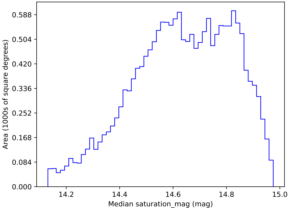
weather_cloudso2v3.4_10yrs WFD r band: Median saturation_mag
