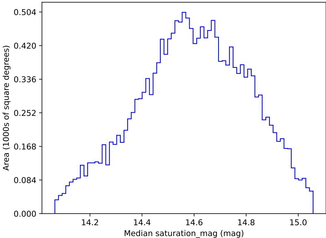
weather_cloudso2v3.4_10yrs WFD g band: Median saturation_mag
