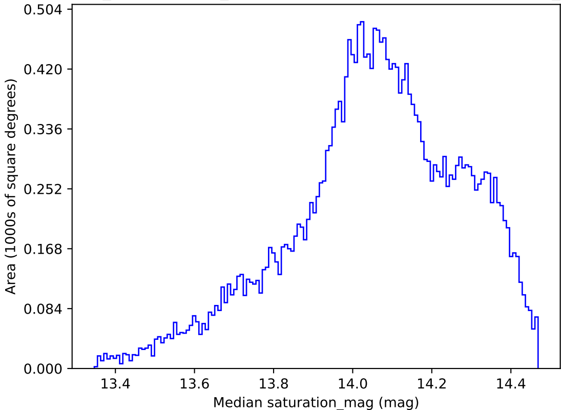
weather_cloudso2v3.4_10yrs All sky z band: Median saturation_mag
