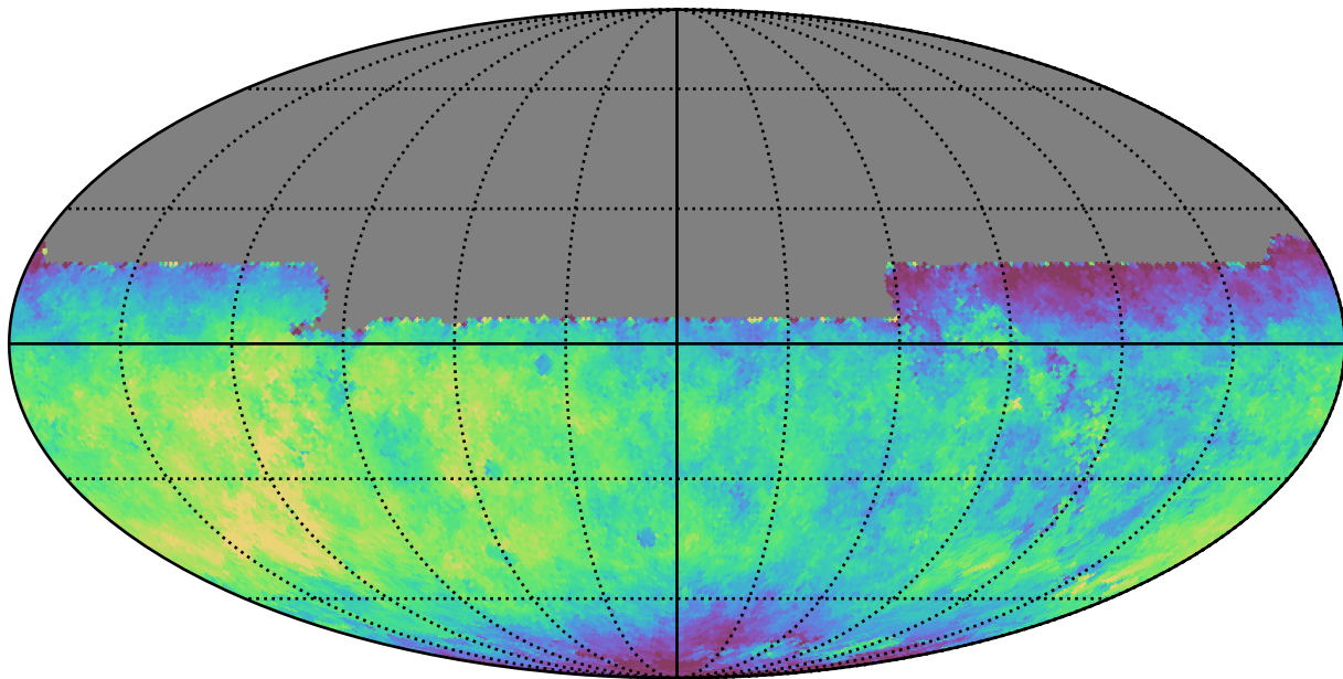
weather_cloudso2v3.4_10yrs All sky y band: Median saturation_mag
