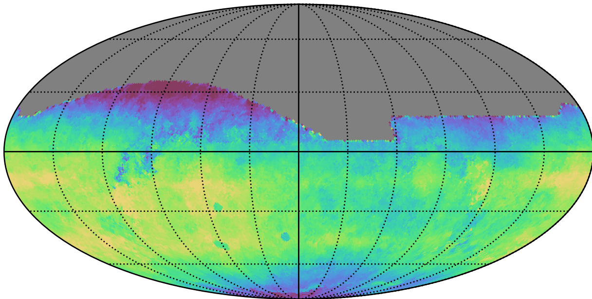
weather_cloudso2v3.4_10yrs All sky r band: Median saturation_mag
