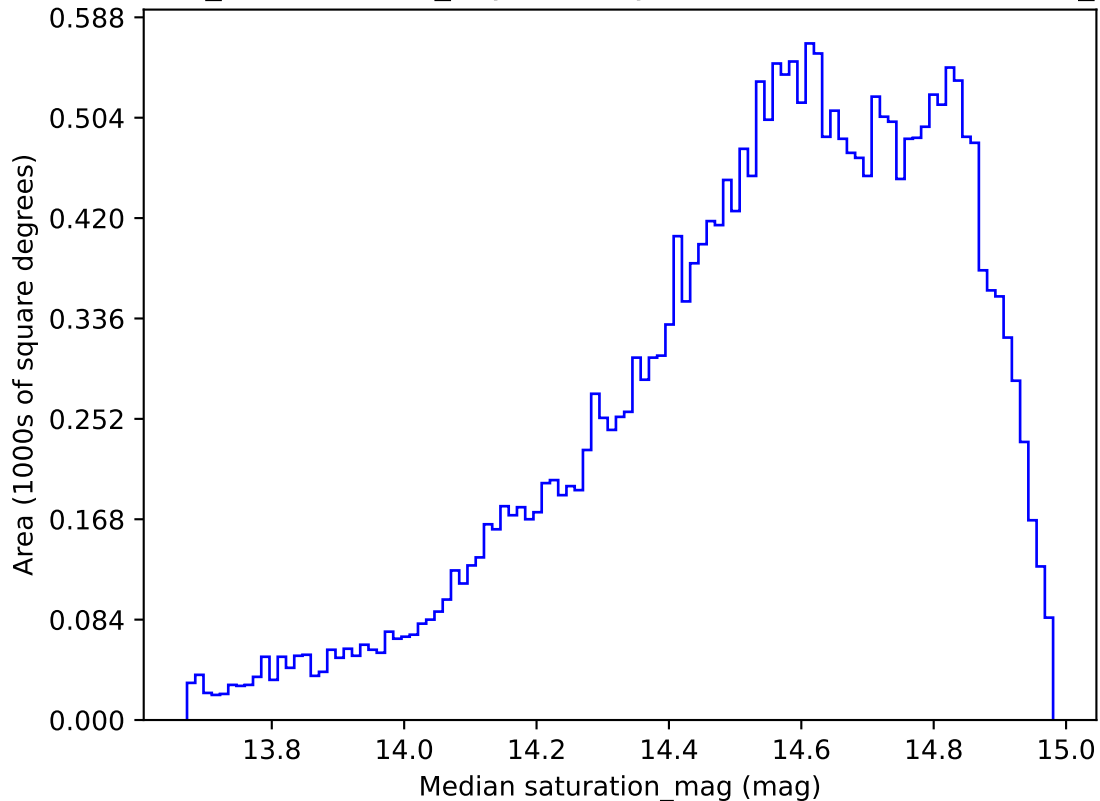
weather_cloudso2v3.4_10yrs All sky r band: Median saturation_mag
