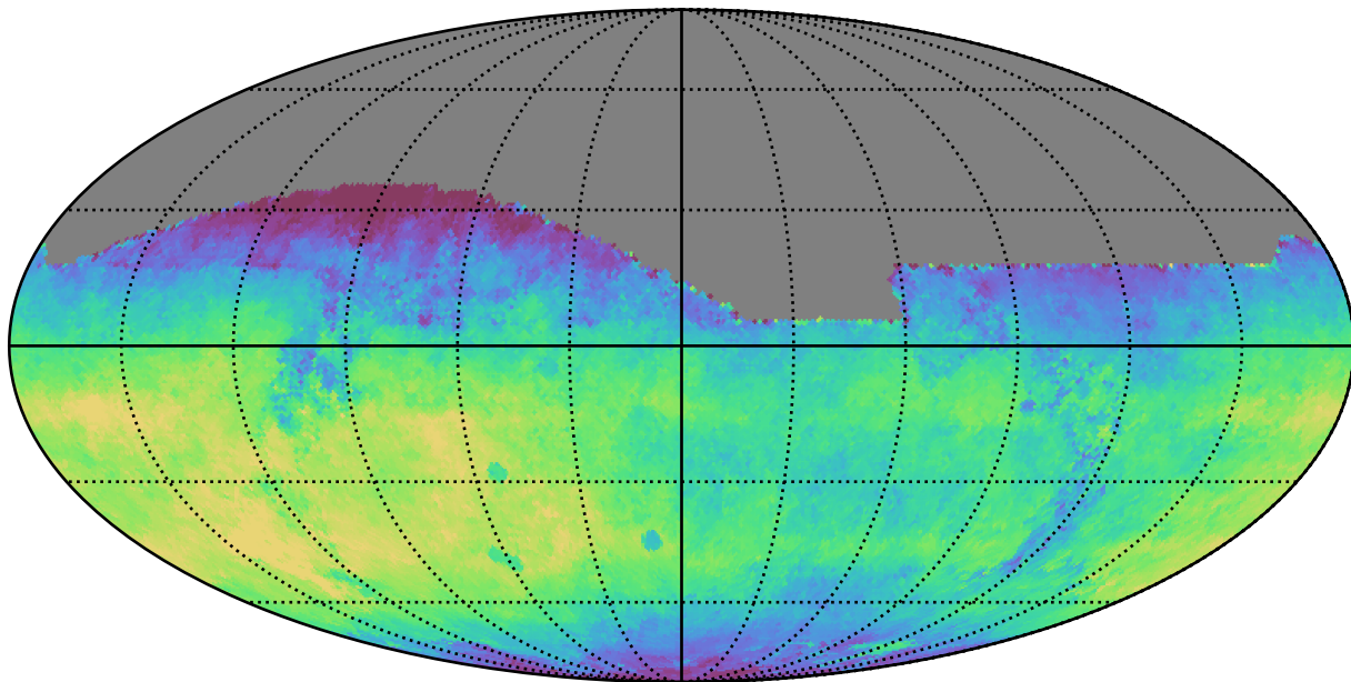
weather_cloudso2v3.4_10yrs All sky i band: Median saturation_mag
