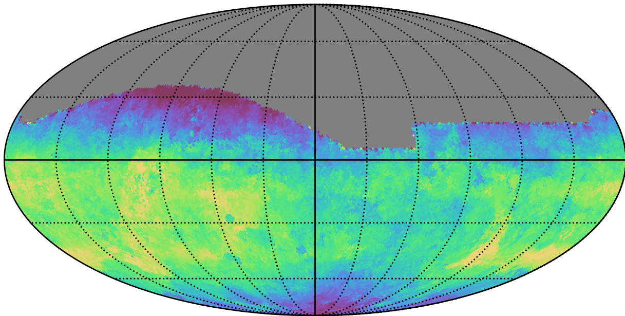
weather_cloudso2v3.4_10yrs All sky g band: Median saturation_mag
