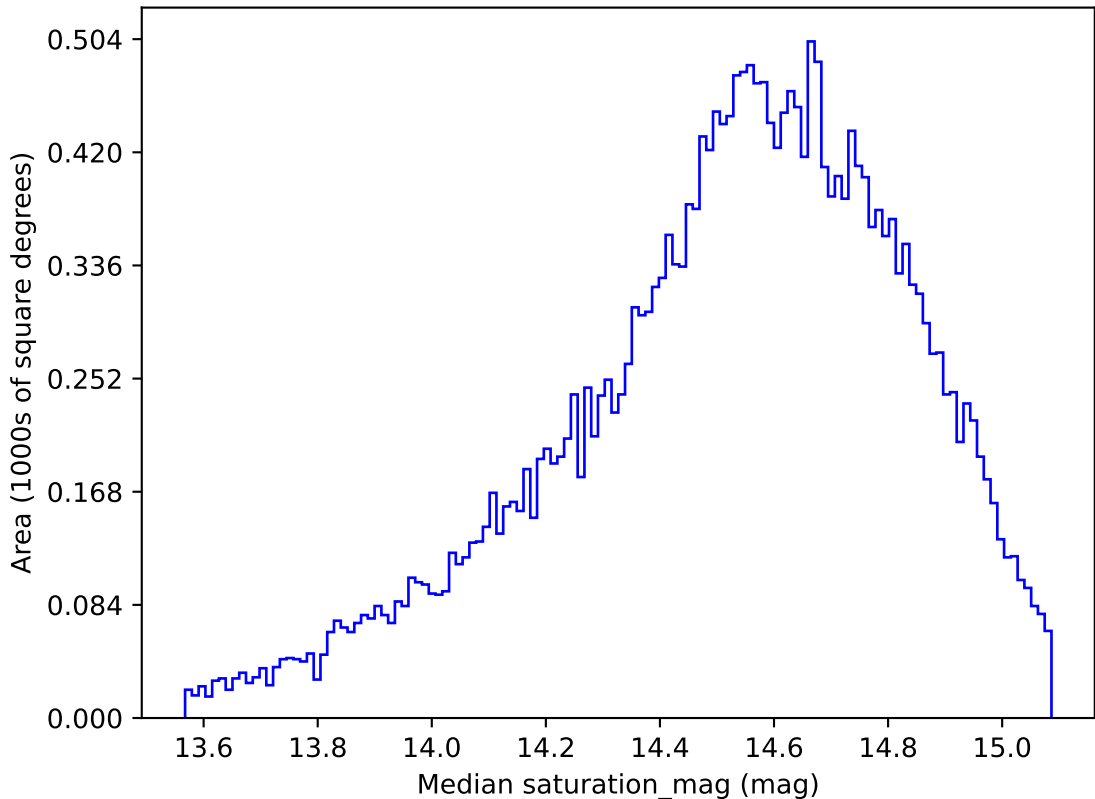
weather_cloudso2v3.4_10yrs All sky g band: Median saturation_mag
