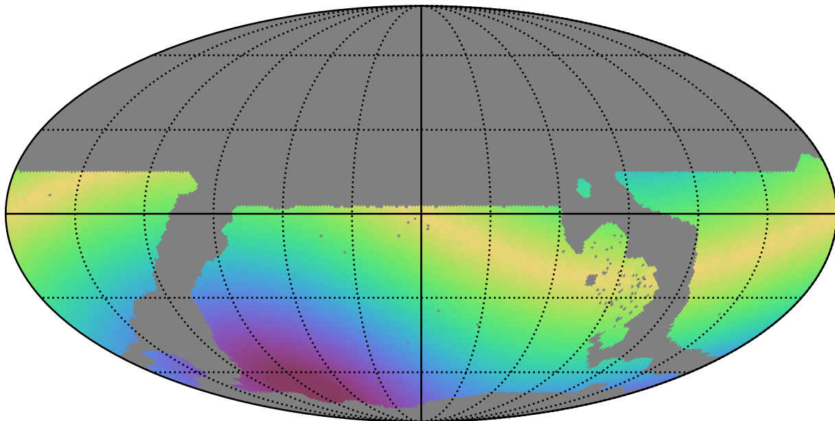
weather_cloudso2v3.4_10yrs WFD y band: Max solarElong
