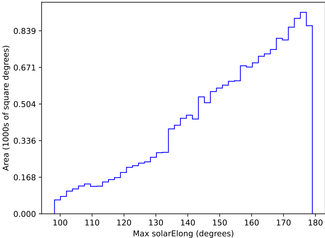
weather_cloudso2v3.4_10yrs WFD g band: Max solarElong
