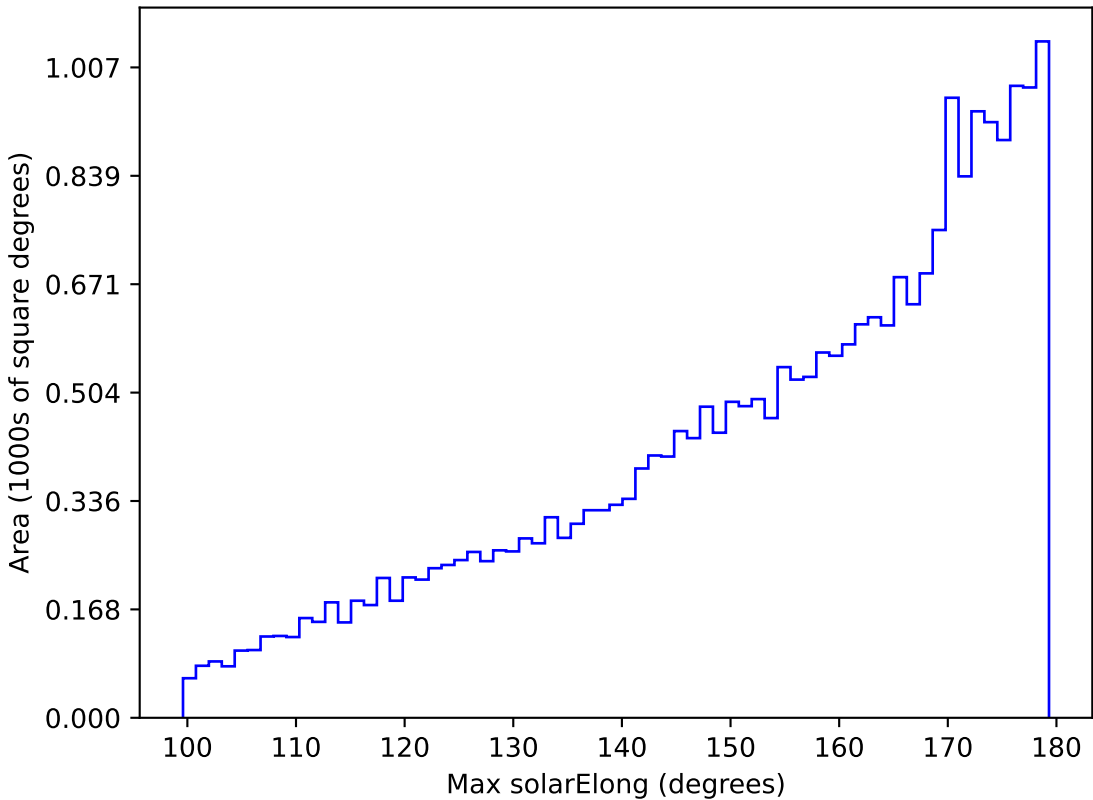
weather_cloudso2v3.4_10yrs All sky z band: Max solarElong
