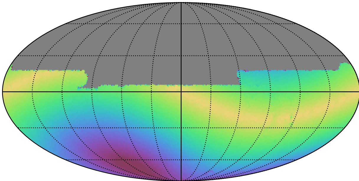
weather_cloudso2v3.4_10yrs All sky y band: Max solarElong
