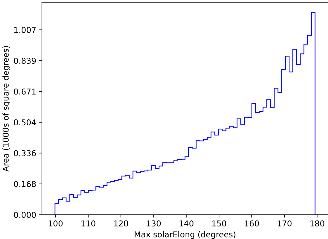
weather_cloudso2v3.4_10yrs All sky i band: Max solarElong
