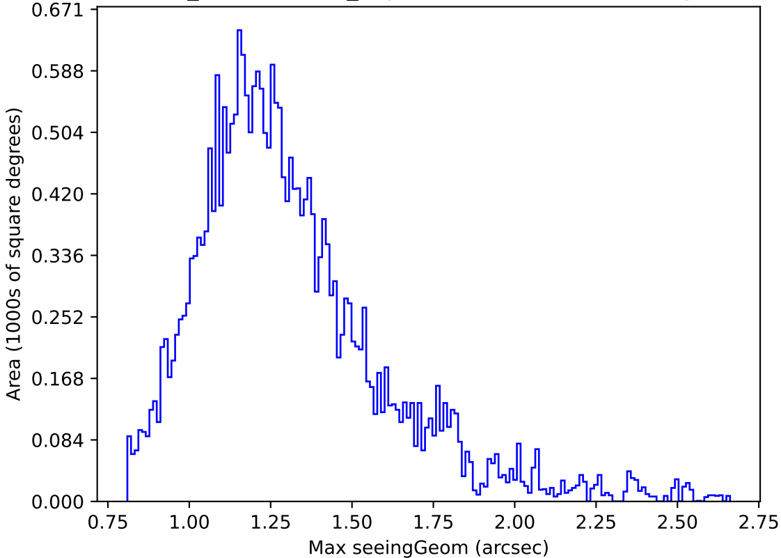
weather_cloudso2v3.4_10yrs Yr 1 z band: Max seeingGeom
