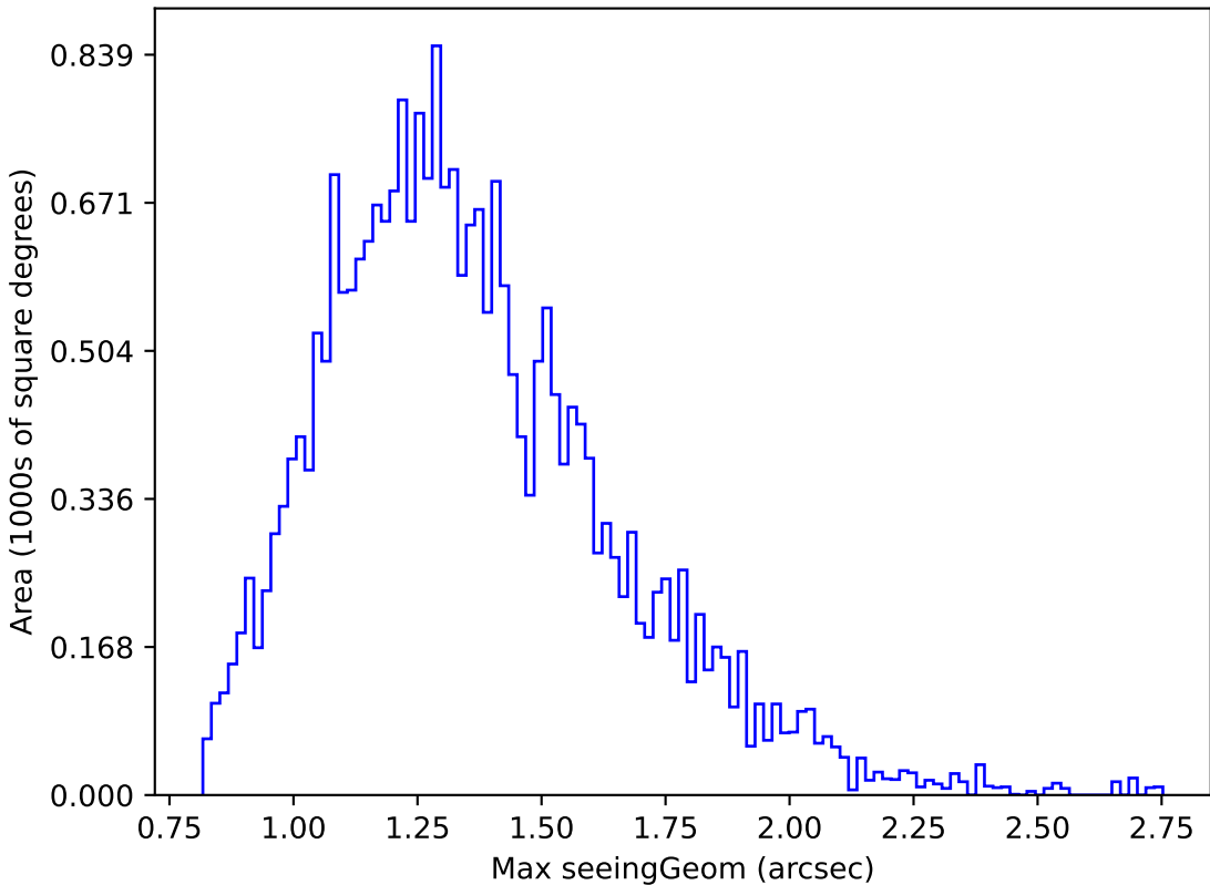
weather_cloudso2v3.4_10yrs Yr 1 r band: Max seeingGeom
