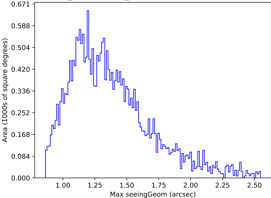
weather_cloudso2v3.4_10yrs Yr 1 i band: Max seeingGeom
