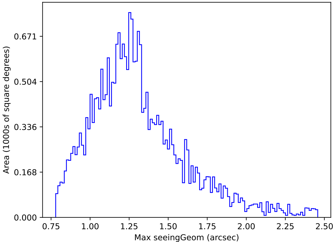
weather_cloudso2v3.4_10yrs Yr 1 g band: Max seeingGeom
