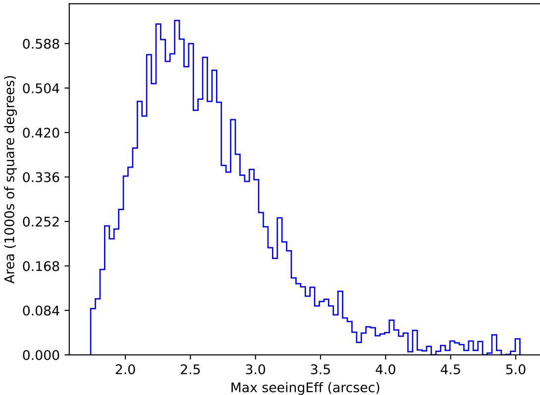
weather_cloudso2v3.4_10yrs WFD z band: Max seeingEff
