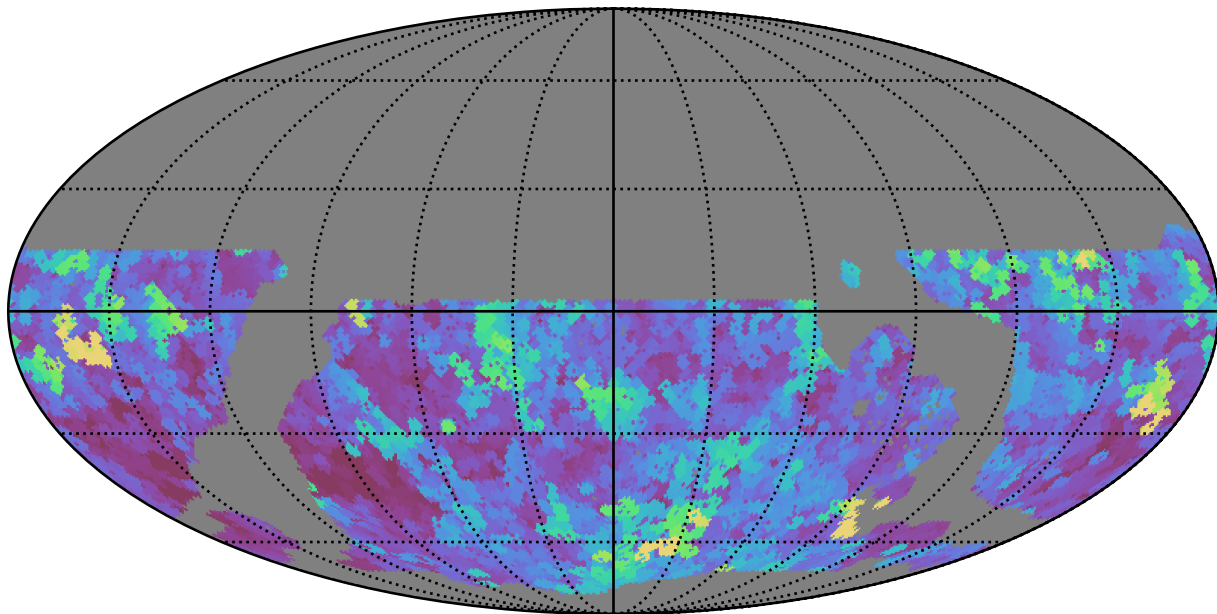
weather_cloudso2v3.4_10yrs WFD i band: Max seeingEff
