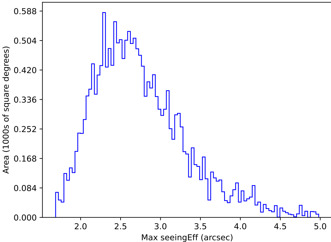
weather_cloudso2v3.4_10yrs WFD i band: Max seeingEff
