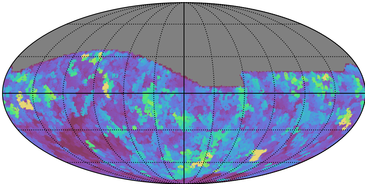
weather_cloudso2v3.4_10yrs All sky i band: Max seeingEff
