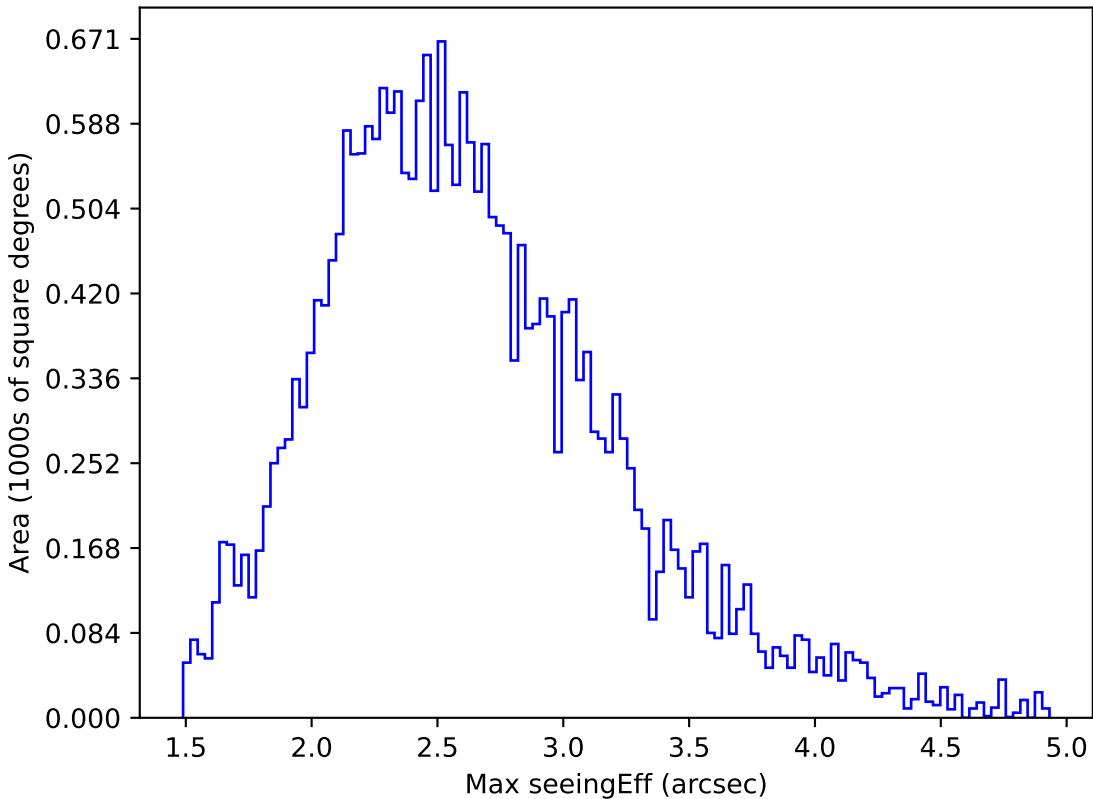
weather_cloudso2v3.4_10yrs All sky i band: Max seeingEff
