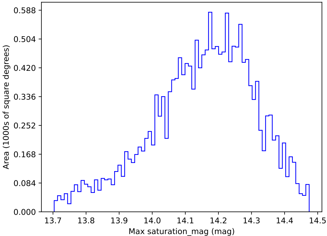
weather_cloudso2v3.4_10yrs WFD y band: Max saturation_mag
