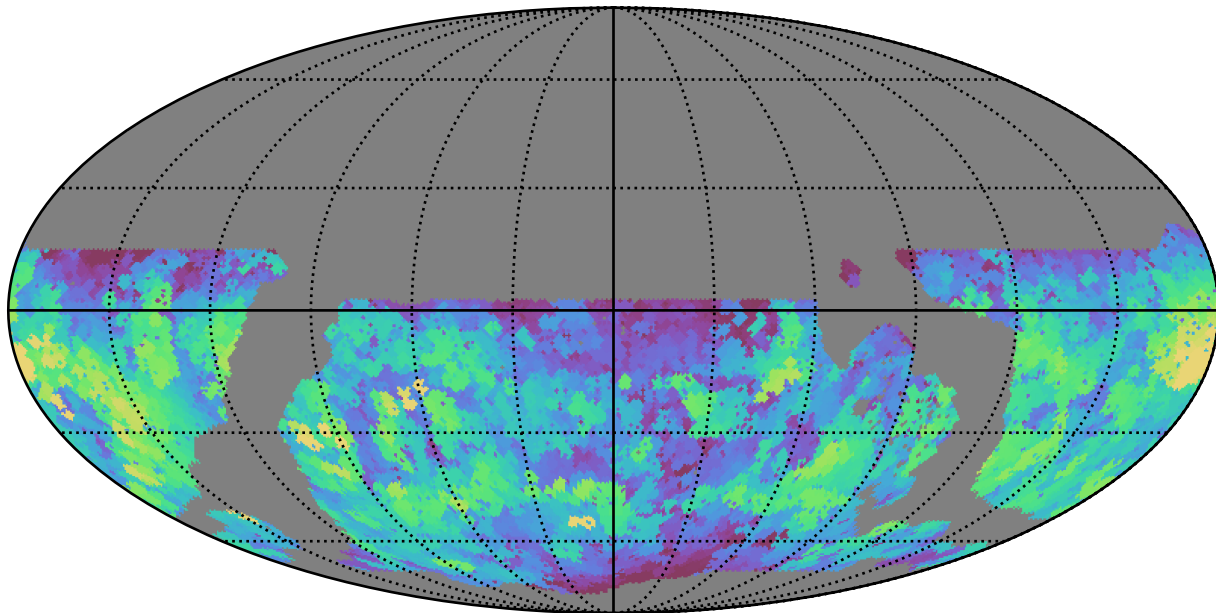
weather_cloudso2v3.4_10yrs WFD u band: Max saturation_mag
