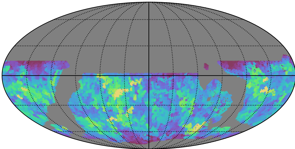
weather_cloudso2v3.4_10yrs WFD r band: Max saturation_mag
