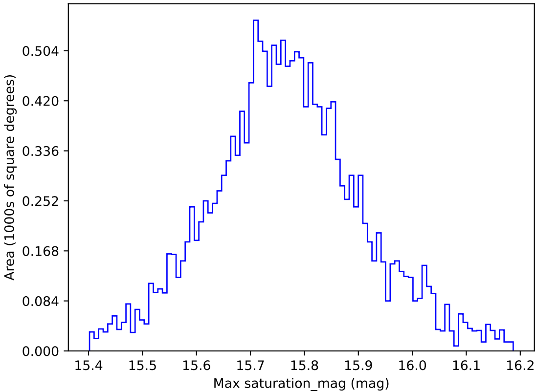
weather_cloudso2v3.4_10yrs WFD r band: Max saturation_mag
