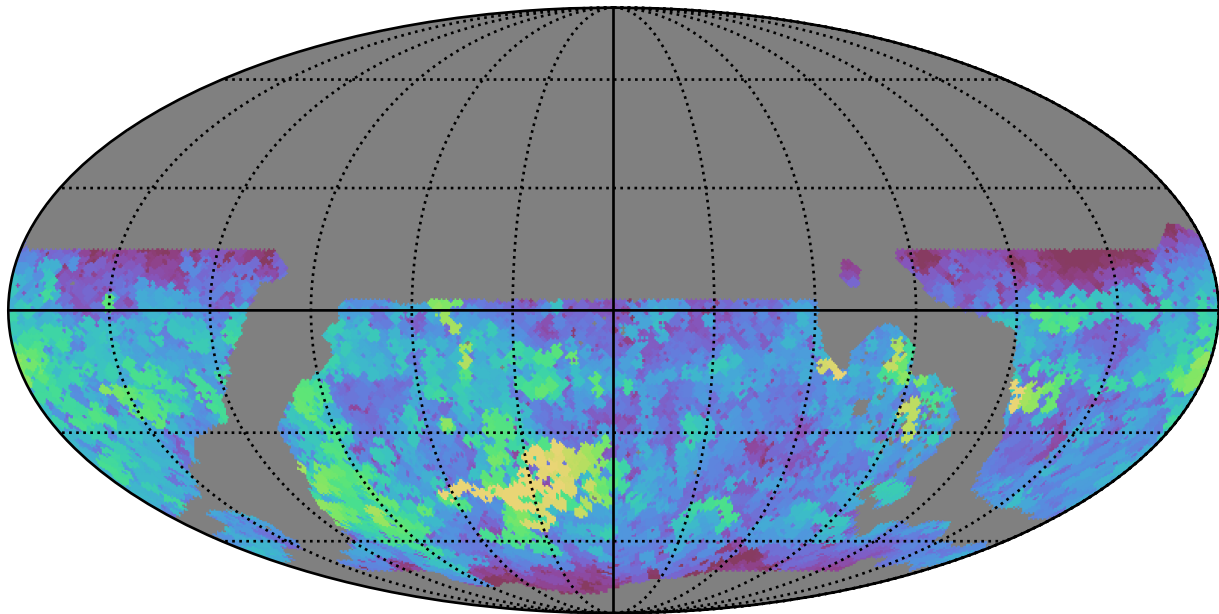
weather_cloudso2v3.4_10yrs WFD g band: Max saturation_mag
