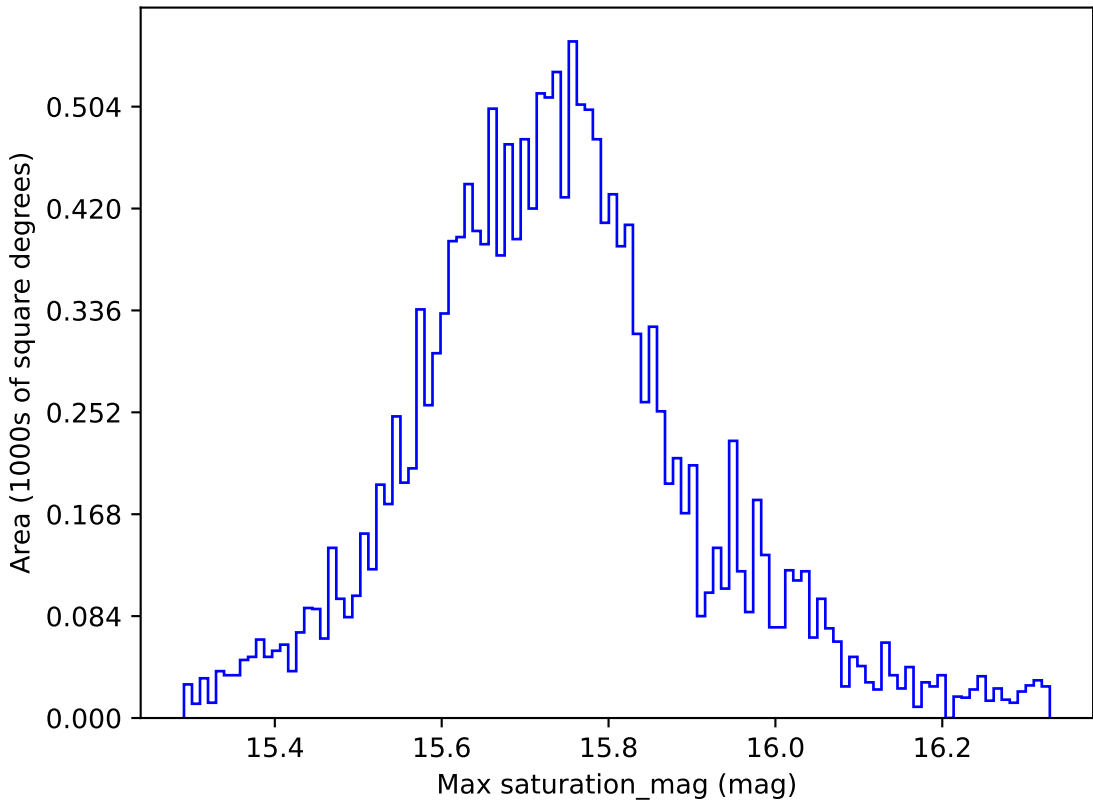
weather_cloudso2v3.4_10yrs WFD g band: Max saturation_mag
