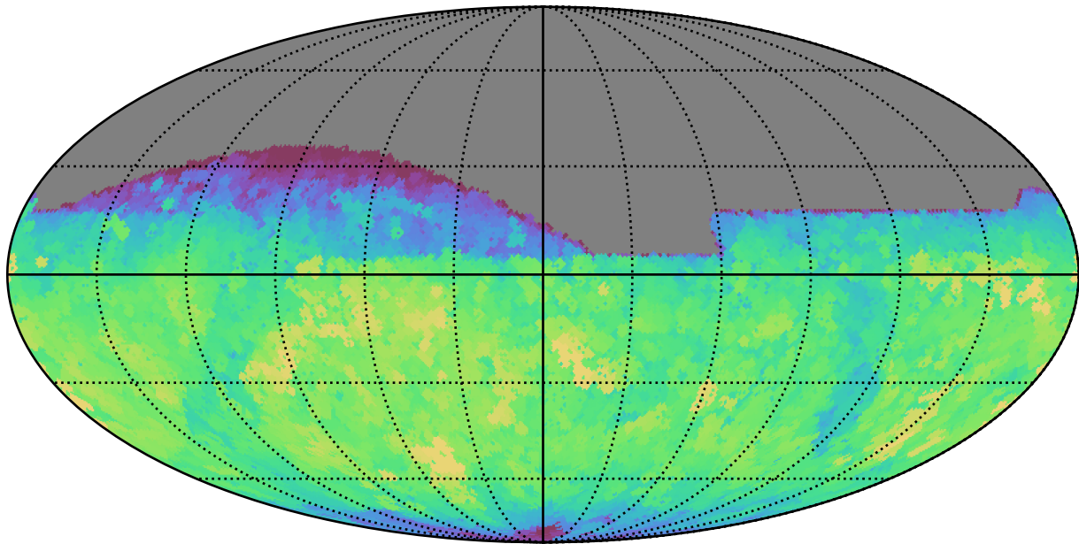
weather_cloudso2v3.4_10yrs All sky z band: Max saturation_mag
