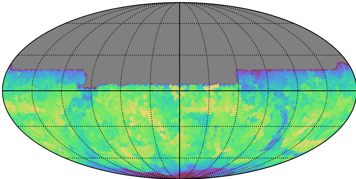
weather_cloudso2v3.4_10yrs All sky y band: Max saturation_mag
