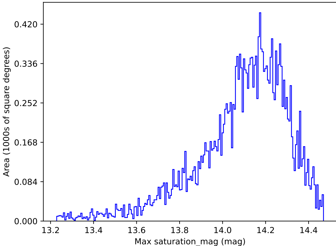
weather_cloudso2v3.4_10yrs All sky y band: Max saturation_mag
