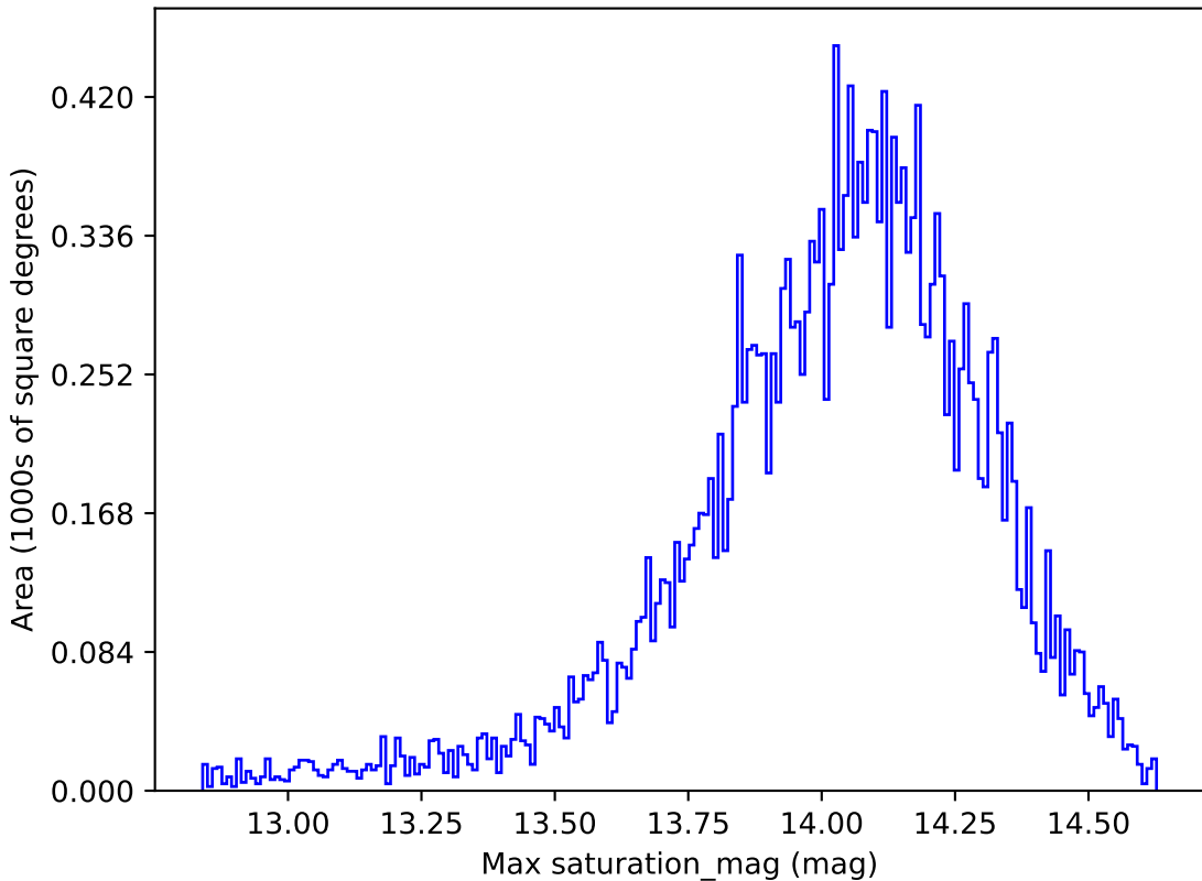
weather_cloudso2v3.4_10yrs All sky u band: Max saturation_mag
