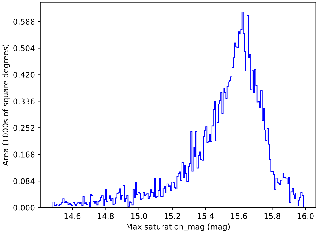
weather_cloudso2v3.4_10yrs All sky i band: Max saturation_mag
