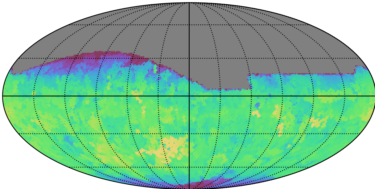
weather_cloudso2v3.4_10yrs All sky g band: Max saturation_mag
