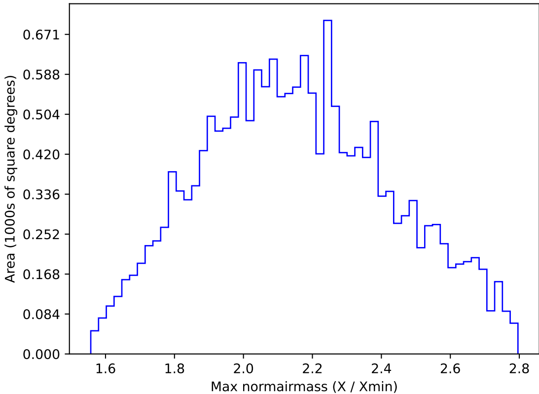
weather_cloudso2v3.4_10yrs WFD y band: Max normairmass
