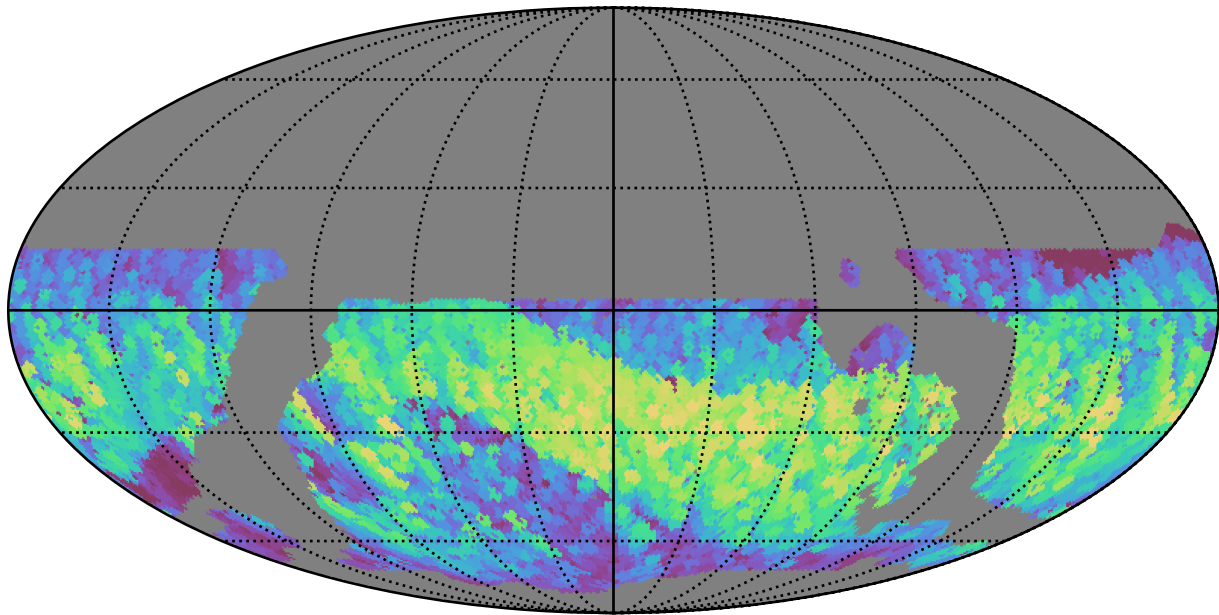
weather_cloudso2v3.4_10yrs WFD i band: Max normairmass
