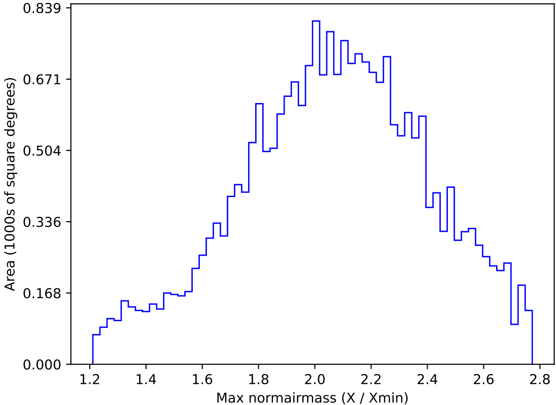
weather_cloudso2v3.4_10yrs All sky y band: Max normairmass
