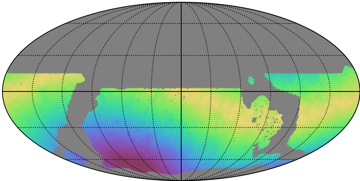
weather_cloudso2v3.4_10yrs WFD z band: Max moonDistance
