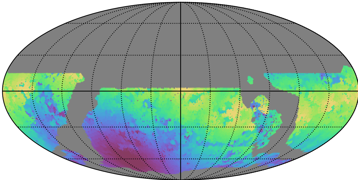
weather_cloudso2v3.4_10yrs WFD y band: Max moonDistance
