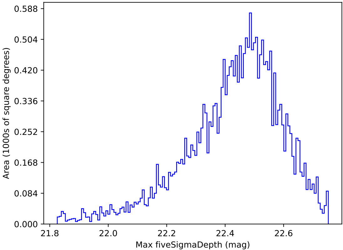
weather_cloudso2v3.4_10yrs Yr 1 y band: Max fiveSigmaDepth
