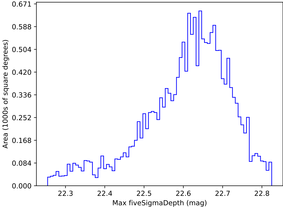
weather_cloudso2v3.4_10yrs WFD y band: Max fiveSigmaDepth
