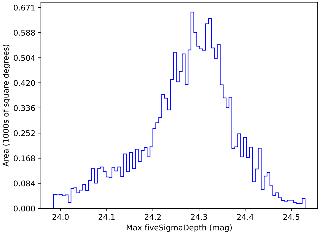
weather_cloudso2v3.4_10yrs WFD i band: Max fiveSigmaDepth
