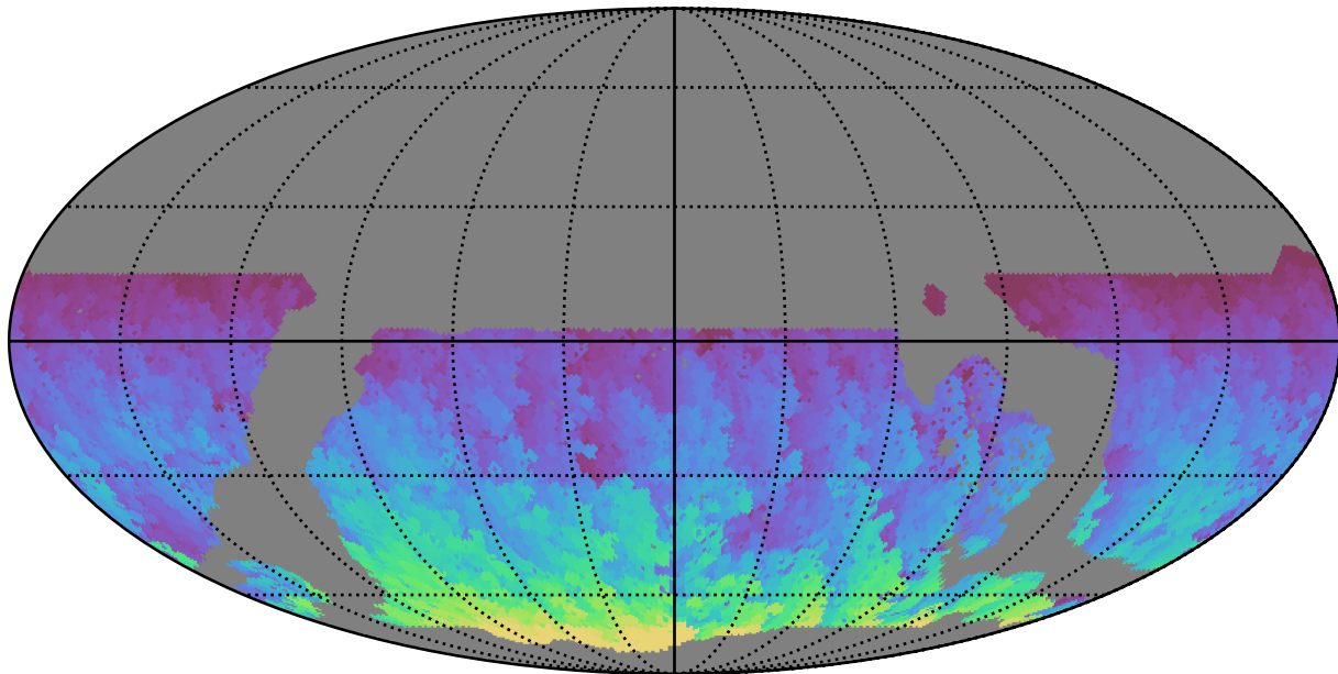
weather_cloudso2v3.4_10yrs WFD y band: Max HA
